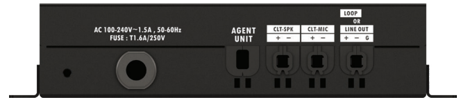
Anschluss-Gerät
